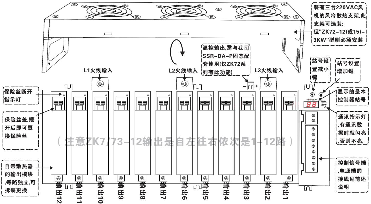
图1:区域功能分布图 (注意ZK7/73-12输出是自左往右依次是1-12路)
