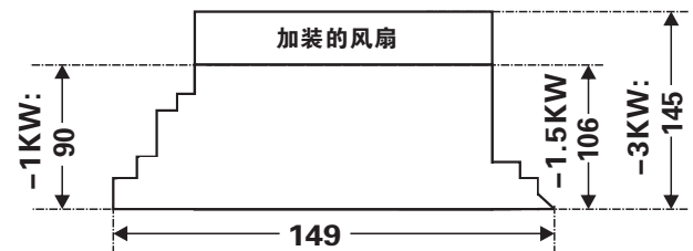
图3:横截面图尺寸
