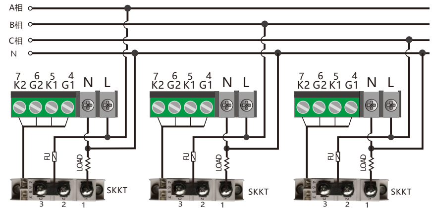
ZKG-Y3电压调整器与SKKT模块三相接线图
