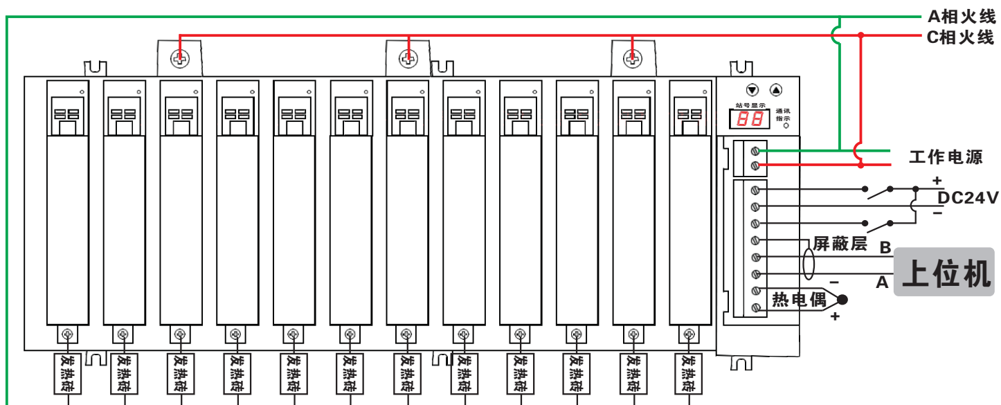
图6.3:三相三线220VAC(C-A相)接线图例
