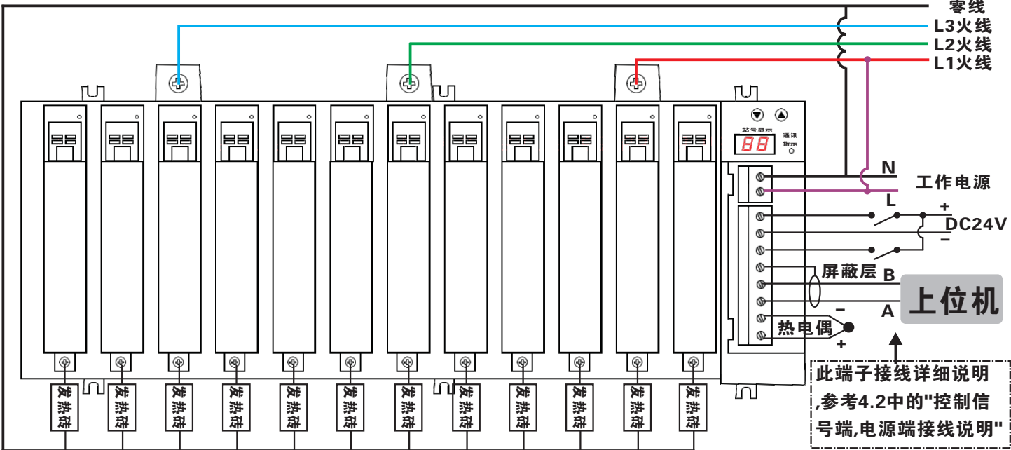
图5:三相四线220VAC接线图例
