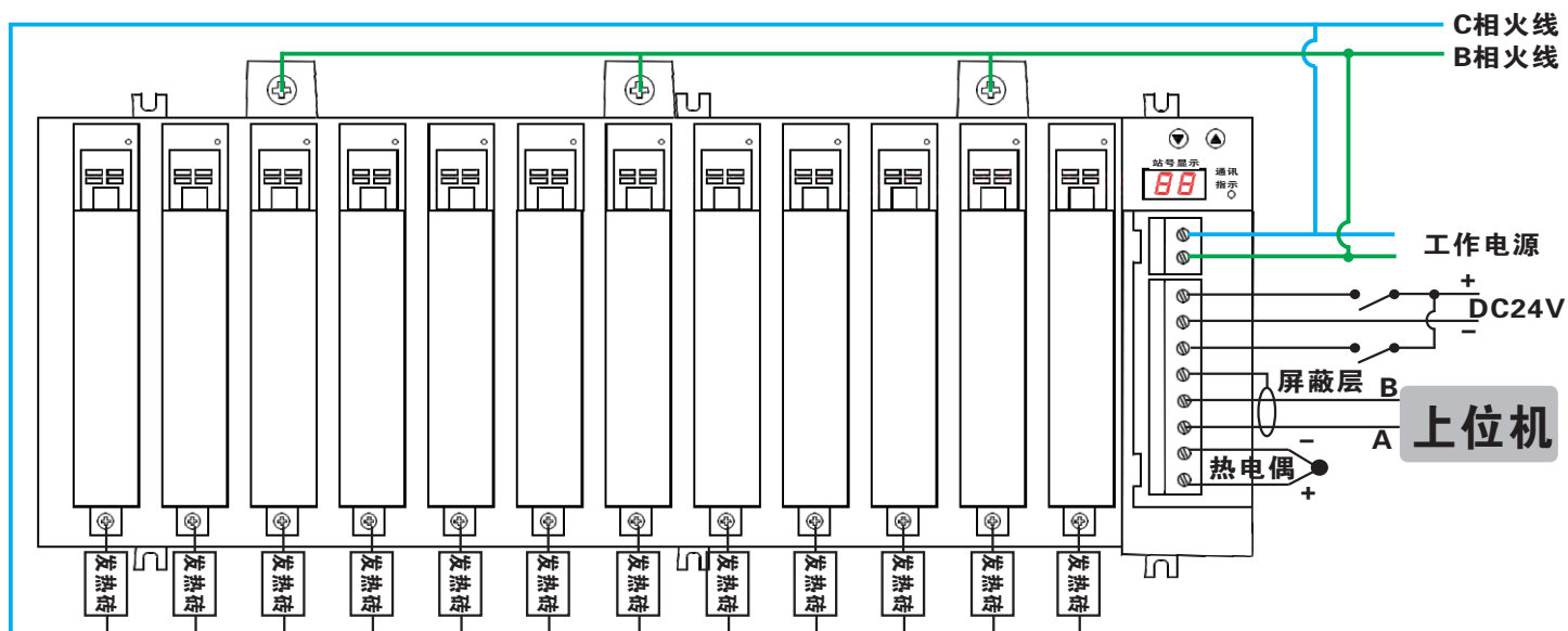
图6.2:三相三线220VAC(B-C相)接线图例
