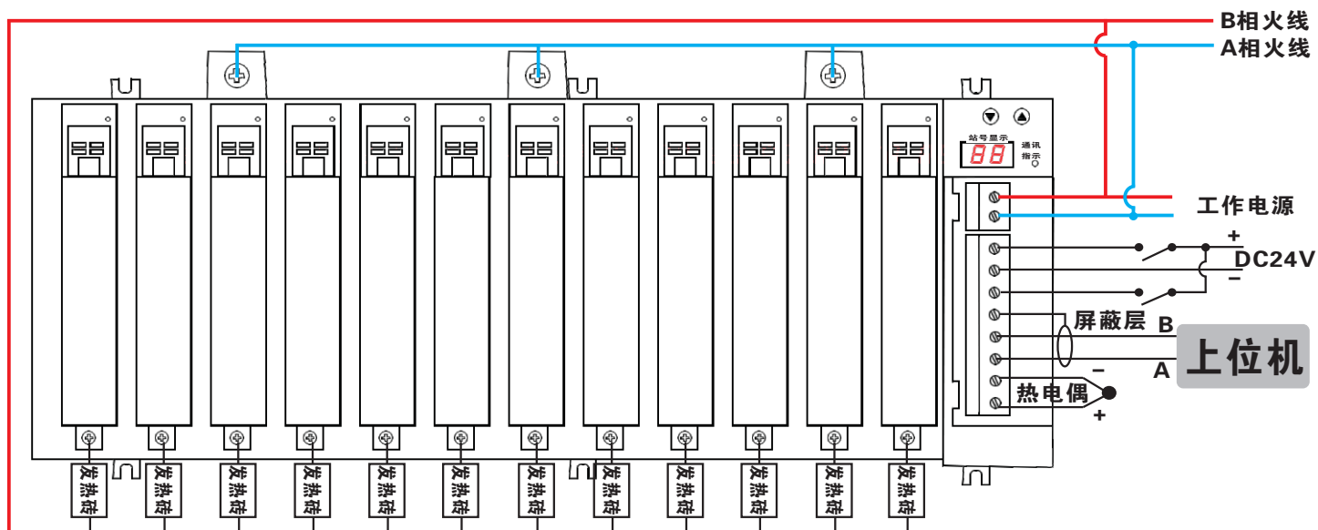
图6.1:三相三线220VAC(A-B相)接线图例
