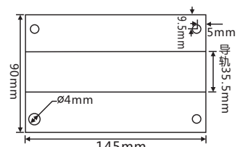
图3：TC-8V4V(-K)类底部装配图
