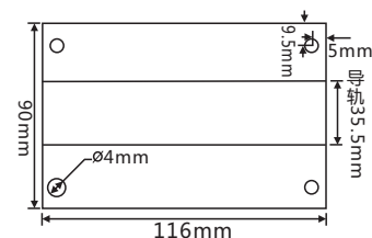
图4：TC-4V4V类底部装配图
